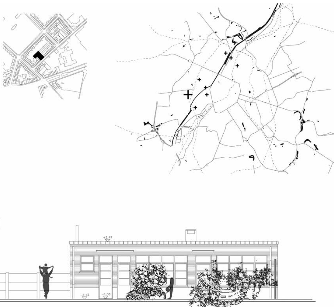
Fig. 3 - Sezione dell'edificio sede del progetto residenziale Le Nid, prima dell'inizio dei lavori. La linea di sezione attraversa il corridoio principale dell'edificio, evidenziando il collegamento diretto tra spazio pubblico e corte interna. La mappa mostra i vari progetti in fase di realizzazione a Bruxelles. Disegno dell'autore. 2018.
