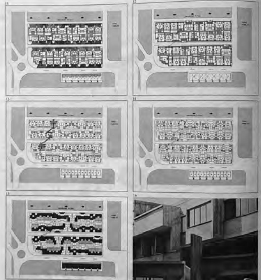
11-15 Grundrisse der angeregten Klappen: Erdgeschoss (11), Hochgeschoss (12) mit Gemeinschaftsräumen (A1-A3), erstes Obergeschoss (13), zweites Obergeschoss (14), Dachgeschoss (15) / plans du secteur étudié: rez-de-chaussée (11), 1 er étage (12), 2 ème étage (13), 3 ème étage (14), plan des escaliers (15) 16. Detail einer vertikalen Verbindung mit Passerelle / détail d'une liaison verticale avec la passerelle 17. Beispiel eines Wohnungstyps / exemple d'un type de logement: 1. Kellergeschoss / sous-sol, 2. Erdgeschoss / rez-de-chaussée, 3. erstes Obergeschoss / 1 er étage, 4. zweites Obergeschoss / 2 ème étage 18. Passerelle, vom Kindergarten passerelle extérieure / le rôle scolaire 19. Detail einer vertikalen Verbindung mit Passerelle / détail d'une liaison verticale avec la passerelle
